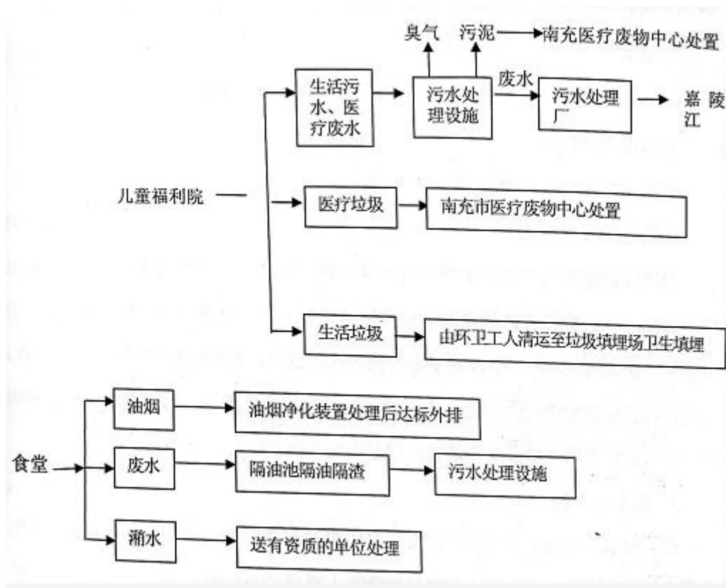
图 2-1-1 儿童福利院工艺流程及产污位置图
